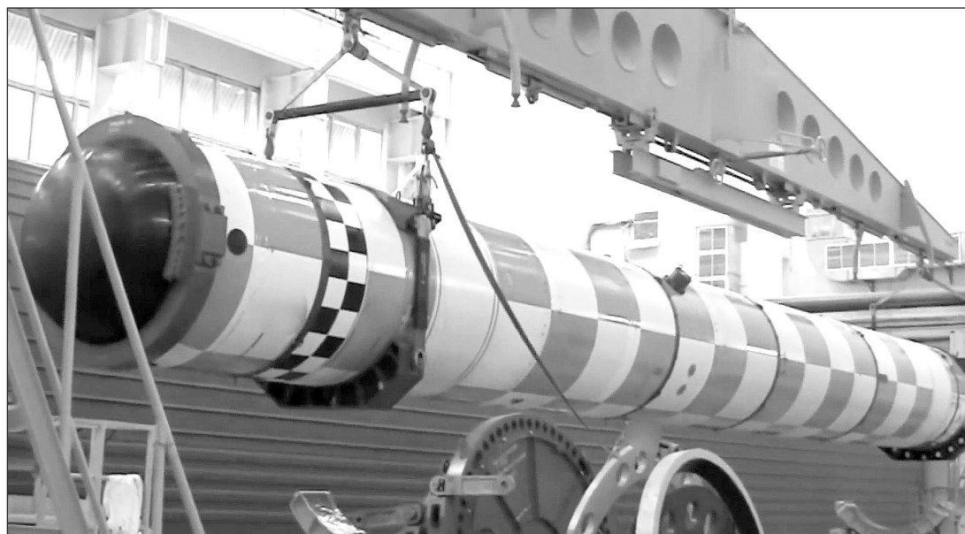
Самодвижущий подводный аппарат 2М39 «Посейдон» на полигонных испытаниях. Кадр видеозаписи Минобороны России.
